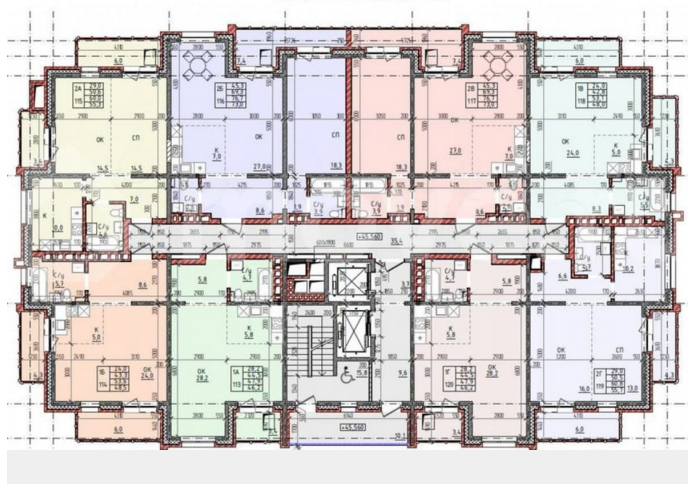
План 16-го этажа на опм. +45,600
